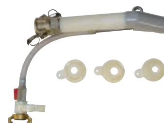
Kit projection 1 lance de projection + 3 buses à projeter Ø 8, Ø 12, Ø 16
